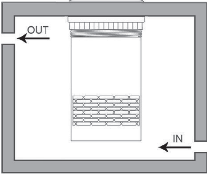
Varias tomas de aire
