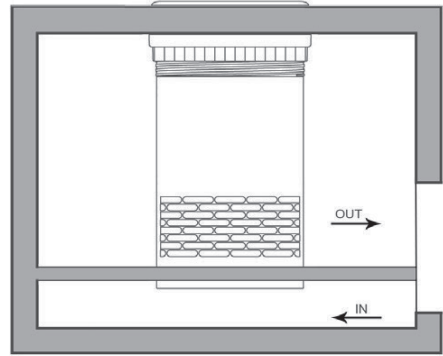
Toma de aire única
